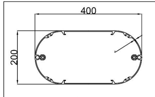
ALT KAİDE PROFİL KESİTİ
