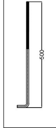
M16 ANKRAJ
