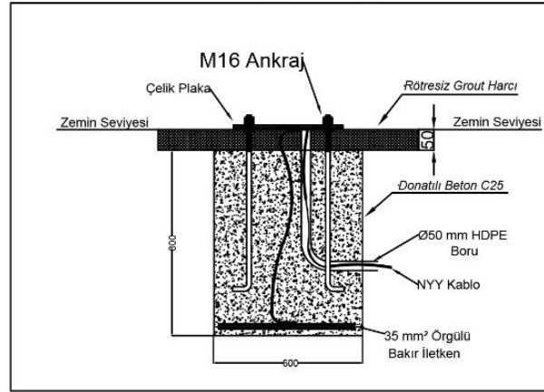
ALT KAİDE PROFİL KESİTİ
